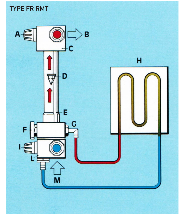
Vor- und Rücklaufkontrolle mit Temperaturerfassung z.B. für Spritzguss
