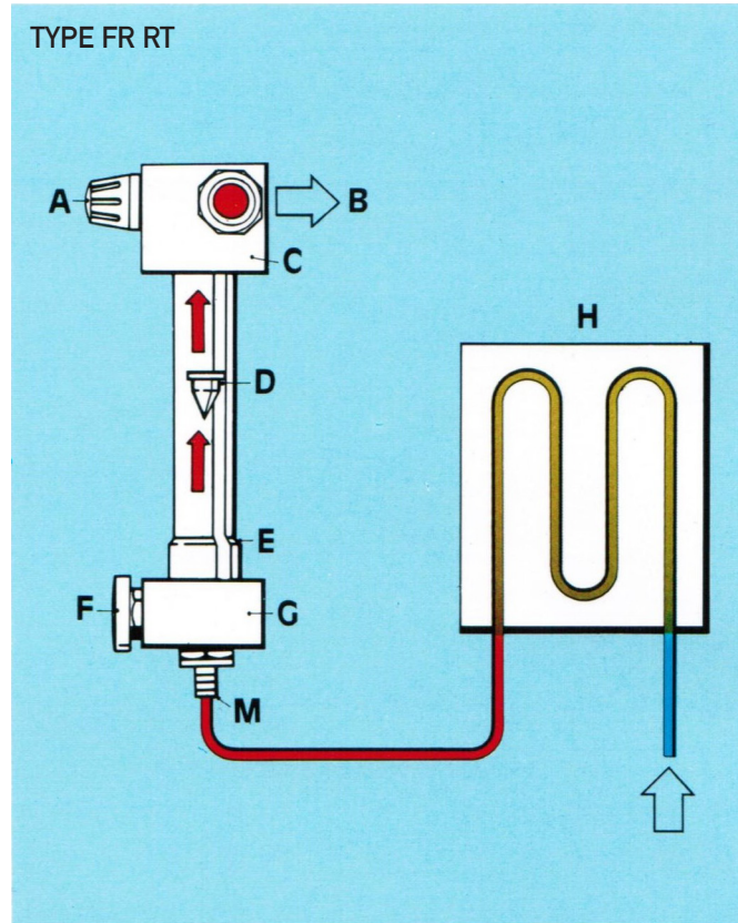
Rücklaufkontrolle mit Temperaturerfassung
