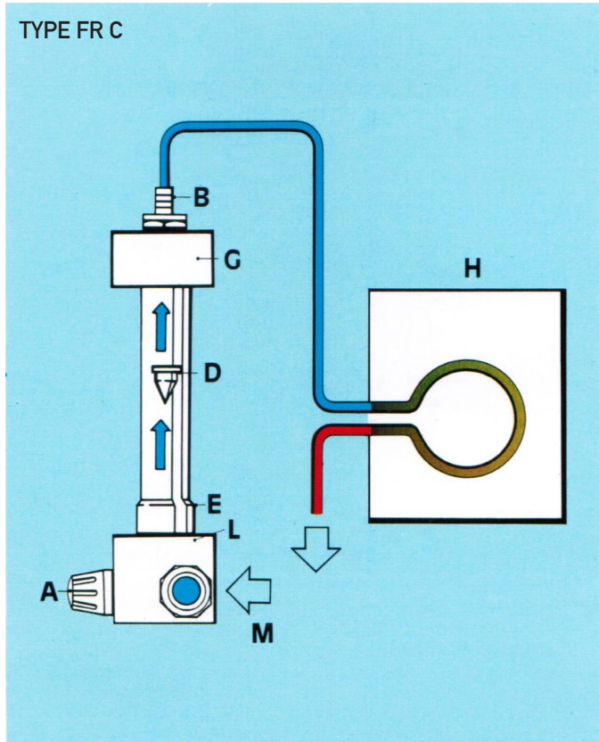
Vorlaufkontrolle z.B. für Druckguss und Extrusion
